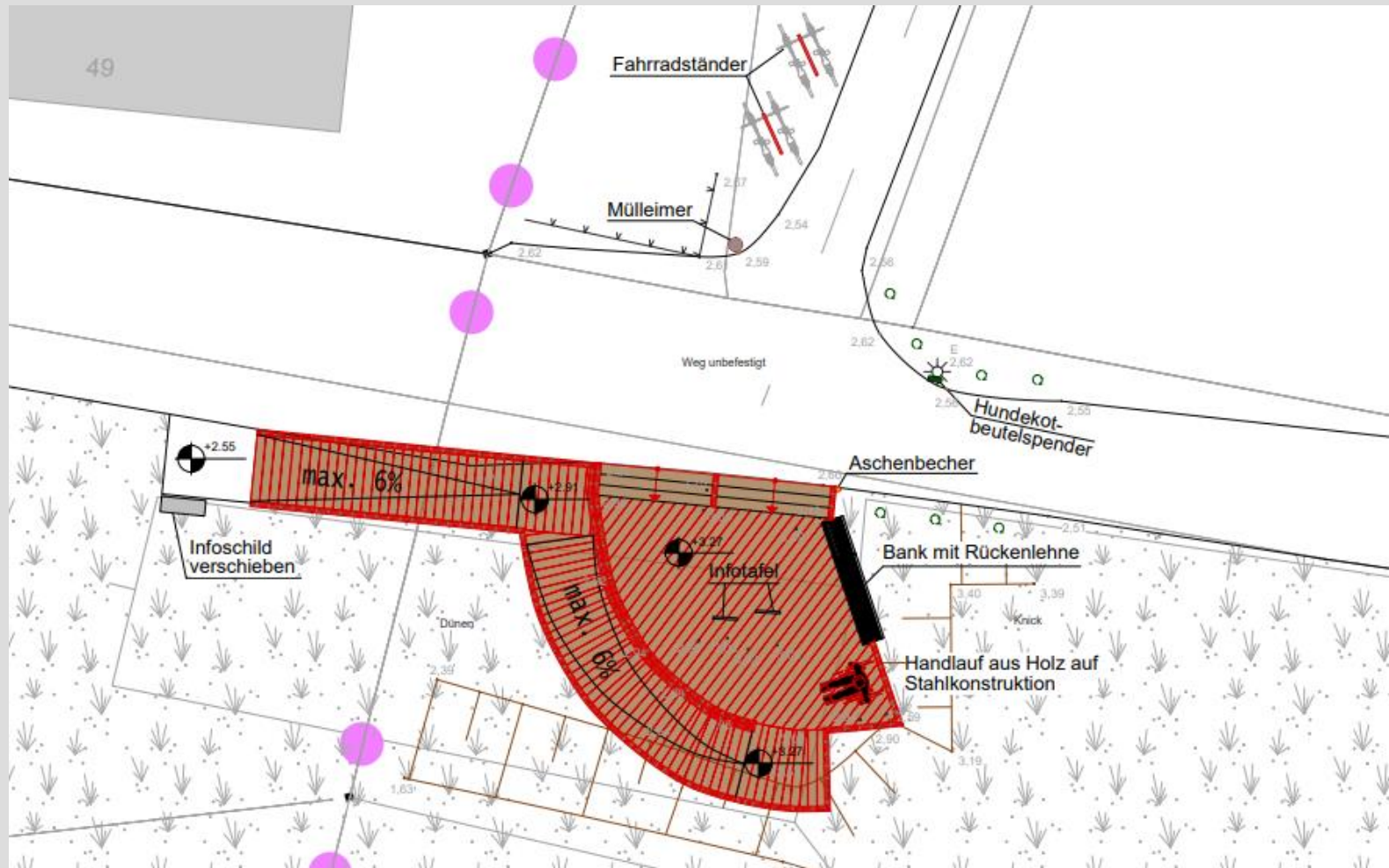
Ruheplatz R1 gemäß Bauplanung
